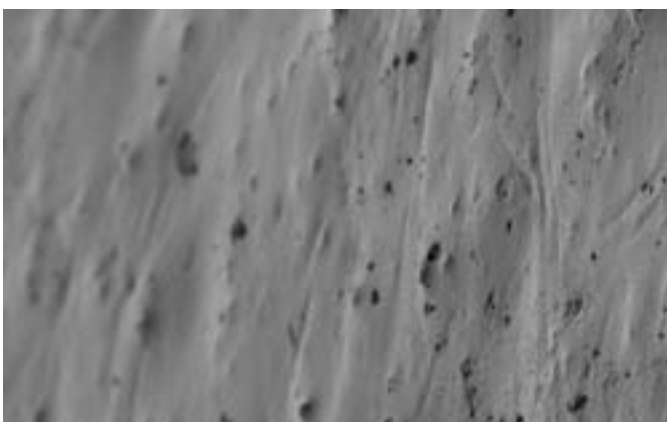
Högtryckslaminat av standardkvalitet. Här ser man tydligt att ytan är betydligt mer ojämn och porig jämfört med laminatet från Dudent. (Förstoring 20 Mμ)
